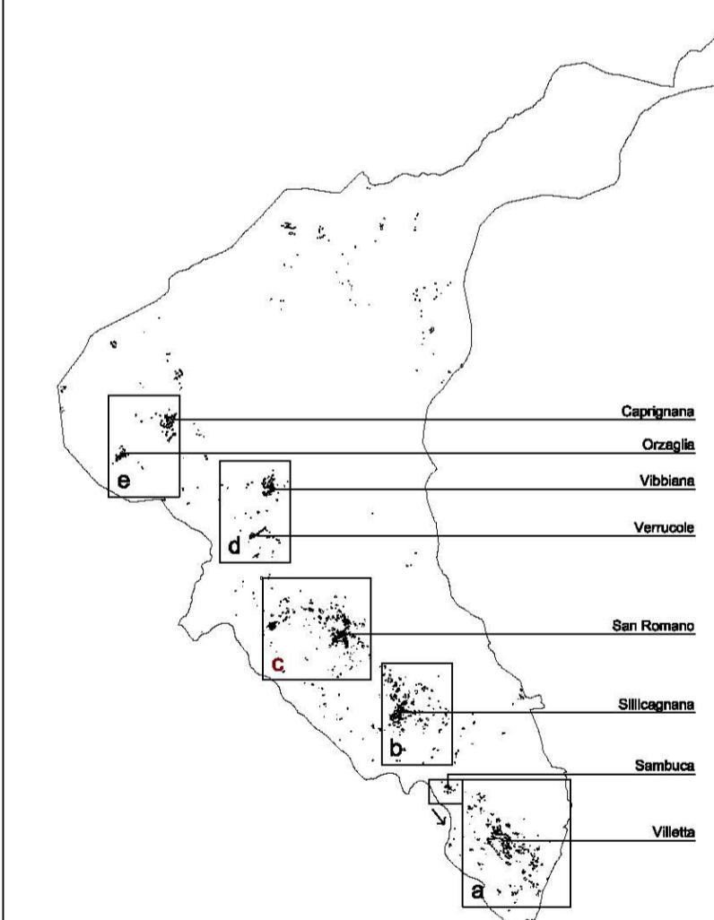
Q3 (b) - Carta delle frequenze fondamentali di risonanza del sottosuolo
