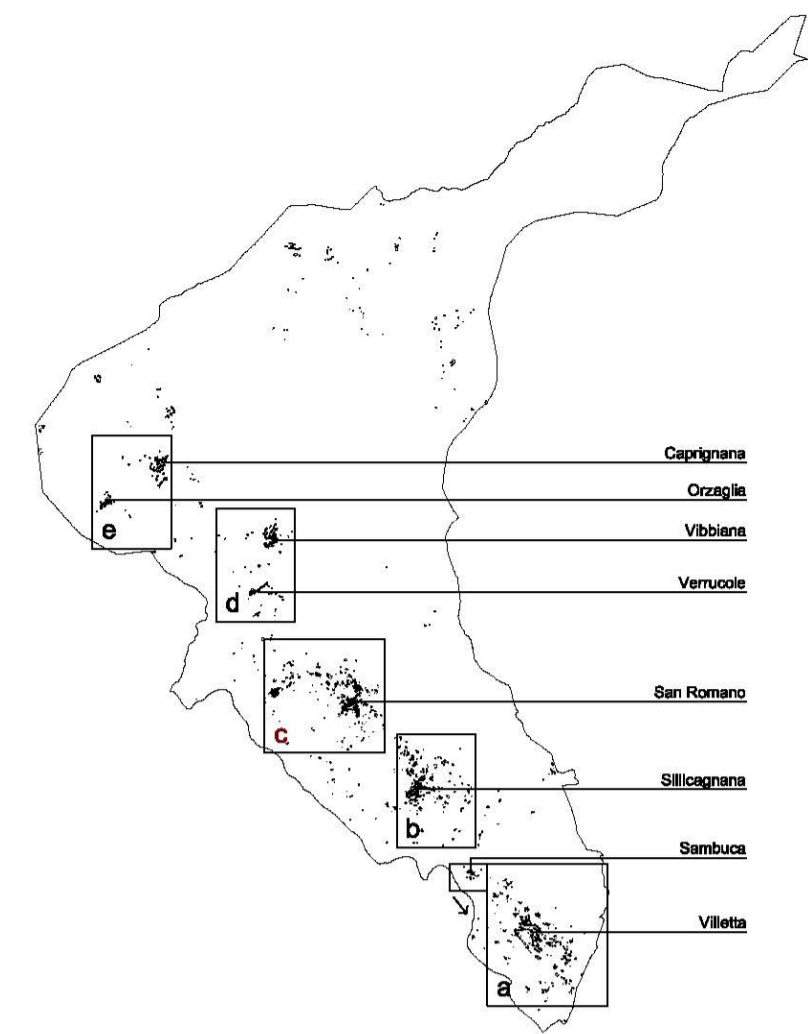
QG3 (d) - Carta delle frequenze fondamentali di risonanza del sottosuolo
