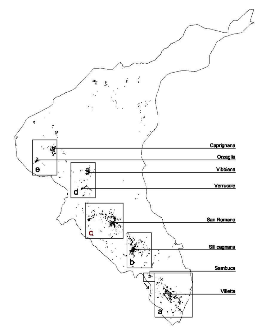
QG3 (e) - Carta delle frequenze fondamentali di risonanza del sottosuolo
