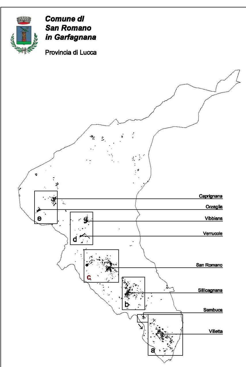
QG1 (a) - Carta geologica e geomorfologica
